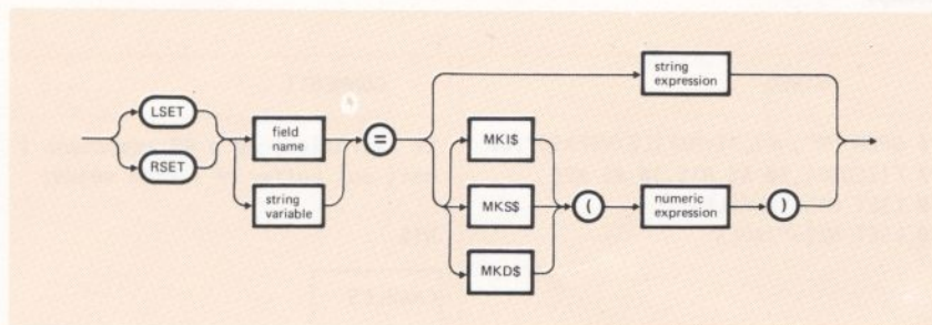
Figura 12-11 Istruzioni LSET/RSET
